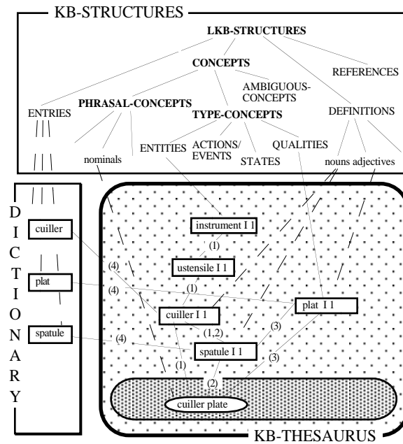
Fig. 1.- The Dictionary Knowledge Base.
